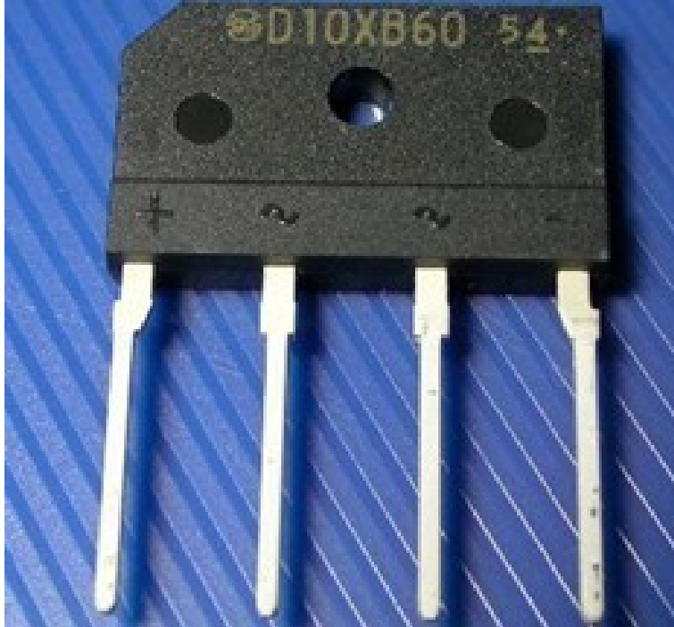
Pont de diodes D10XB60 600V 10A
