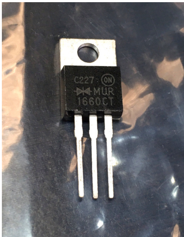
Double diode fast MUR1660CT cathode commune 600V 16A
