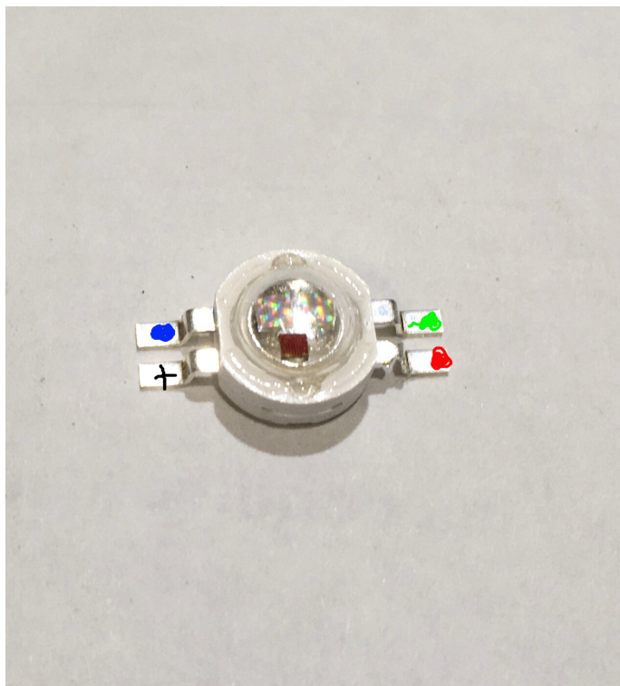
Led RGB à souder en surface 3W 4 pins
