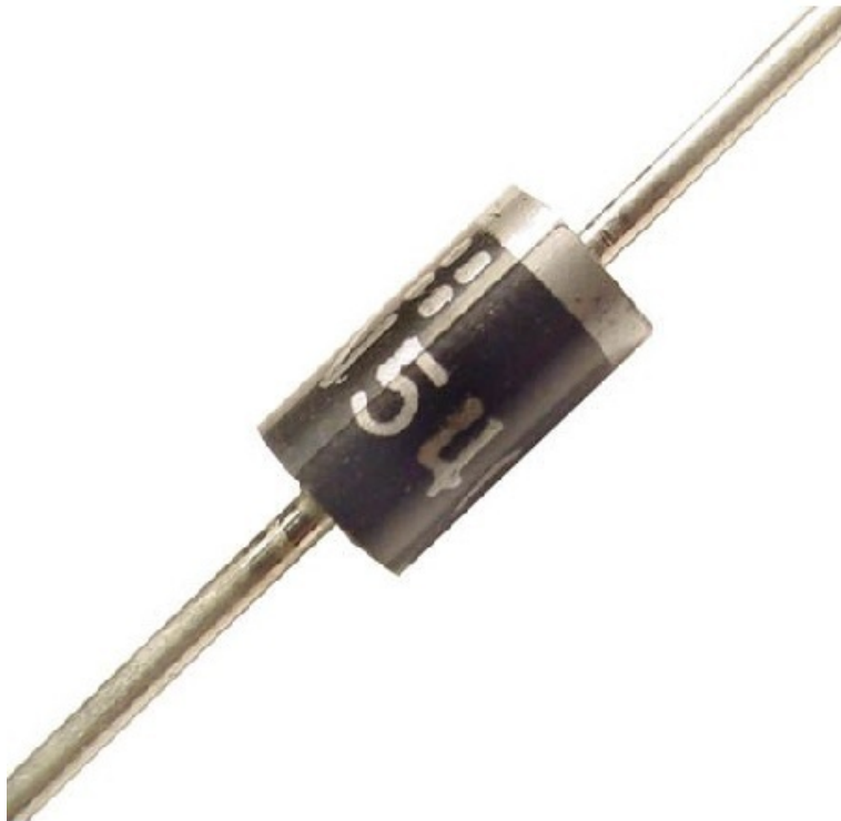
Diode 1N5378B Zener 100V 5W DO201
