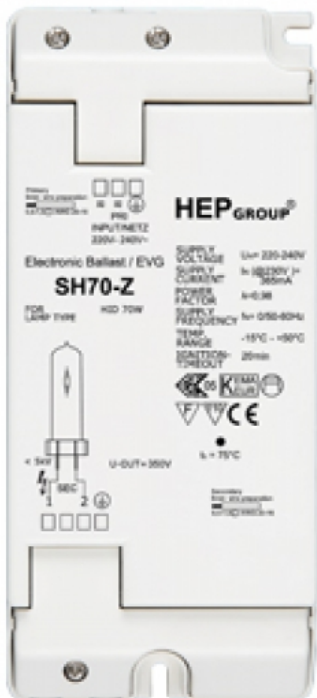
Platine électronique pour lampe à iodure 70W
