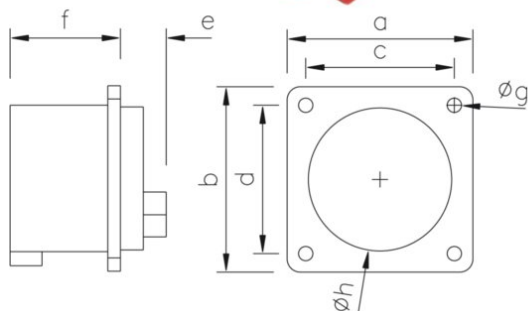
Embase P17 male 16A tétrapolaire 5 broches IP44 Standard à vis
