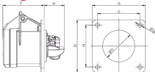
Embase P17 femelle 16A tétrapolaire 5 broches IP44 Turbo Twist
