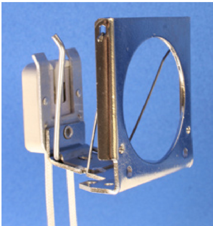
Douille GX5.3 - GY5.3 - GU5.3 avec support MR16
