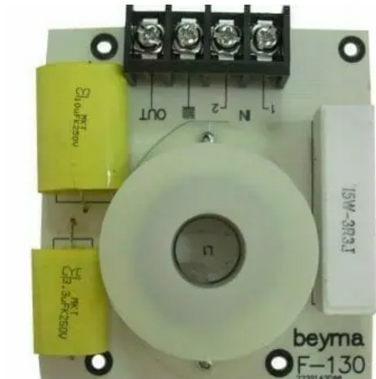
F130 Beyma - Filtre passif passe haut 3KHz
