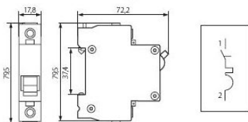
Disjoncteur monophasé 10A courbe B
