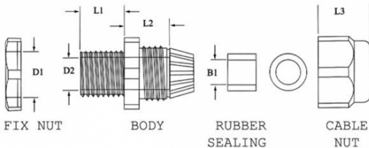
Presse étoupe MG25 pour passage câble de 13 à 18mm
